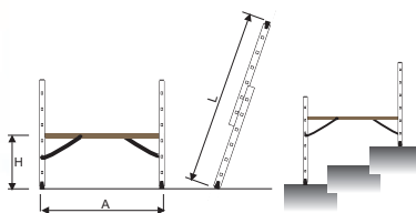
Configurazione scala
